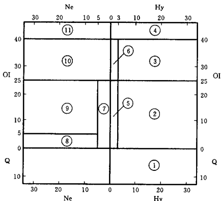
图 15 玄武岩类岩石的 CIPW 标准矿物命名图(OQNH 图)
