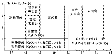
图 12 高镁火山岩(苦橄岩、科马提岩、麦美奇岩和玻古安山岩)的分类和命名
