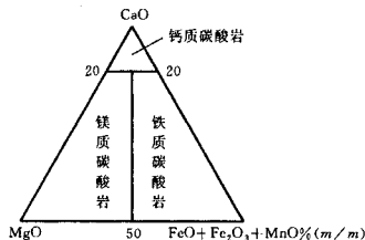
图 3 碳酸岩化学分类和命名
