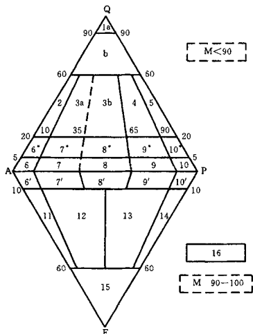
图 5 QAPF 图解的分区分号
