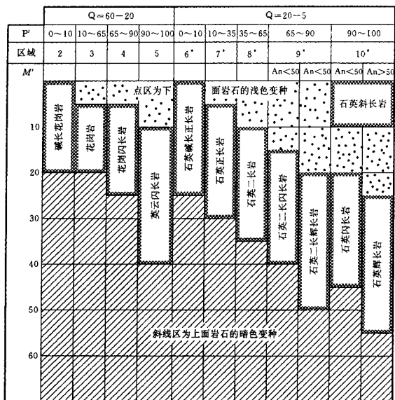
图 7a QAPF 图解(Q>5%)中浅色和暗色岩石变种的 M' = 颜色指数; An = 斜长石牌号
