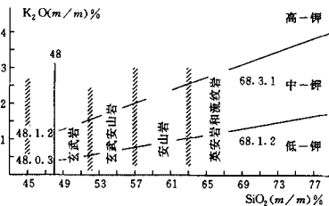
图 16 玄武岩类( SiO_2 > 48\% ),玄武安山岩类、安山岩类、英安岩类和流纹岩类的低钾、中钾和高钾的划分
