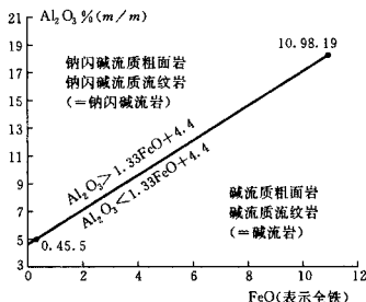
图 17 Al_2O_3 -FeO(全铁)图解
