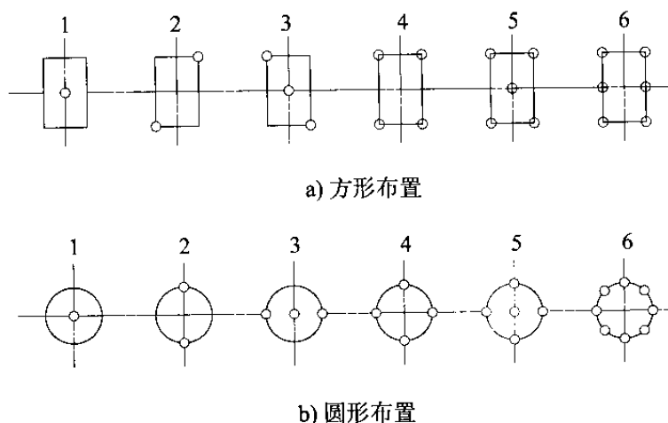
图 6.11.3 勘探钻孔布置图
